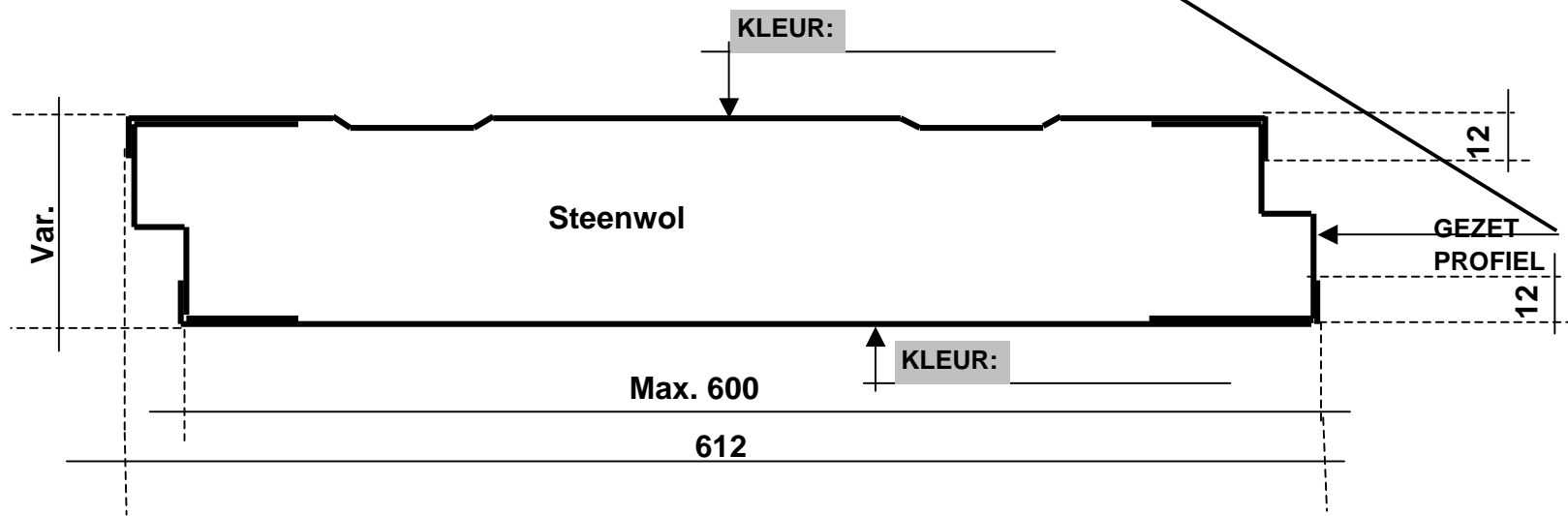
DETAIL GEZET PROFIEL
