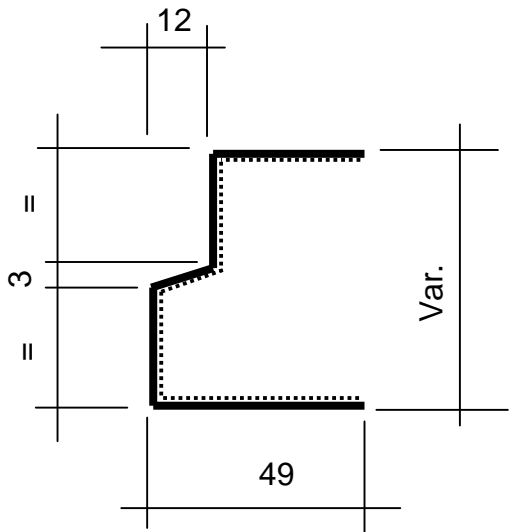
DETAIL GEZET PROFIEL
