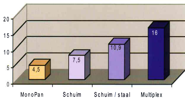
Gewichtsvergelijking (kg/m 2 )
